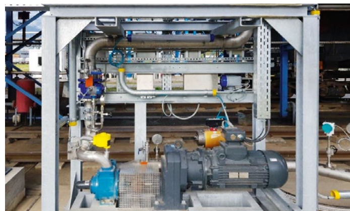
Einlagerungs Pumpe – Skid von INRAG
